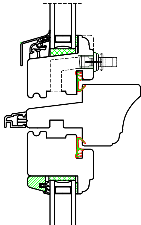
Ventil skjult i bundramme - tværpøst 7.5 A5
