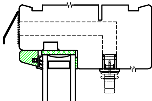
Ventil i topkarm - med vandnæse 7.5 A4
