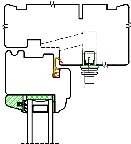
Ventil i topramme - med vandnæse 7.5 A1
