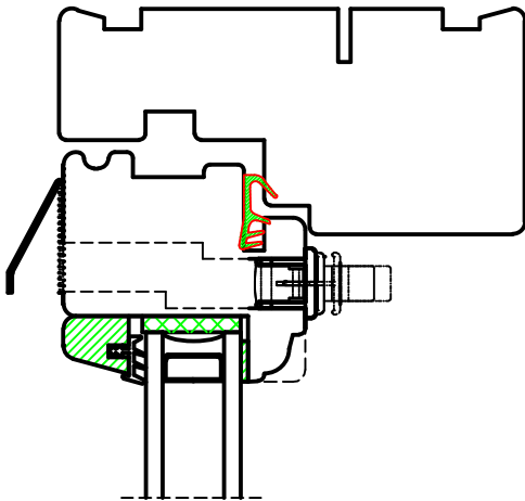
Ventil i topramme - med vandnæse 7.5 A1
