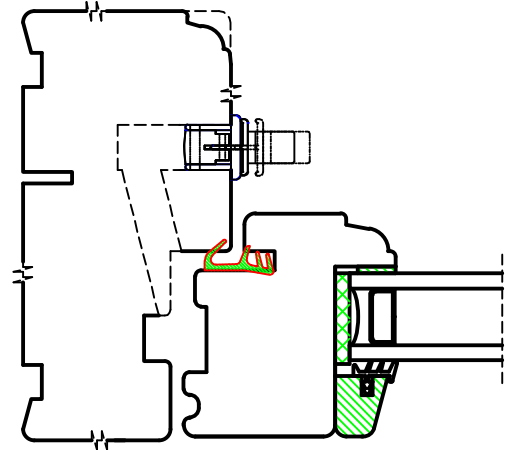
Ventil skjult i sidekarm 7.5 A3
